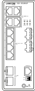
V D LANCOM IGS-3510XUP
