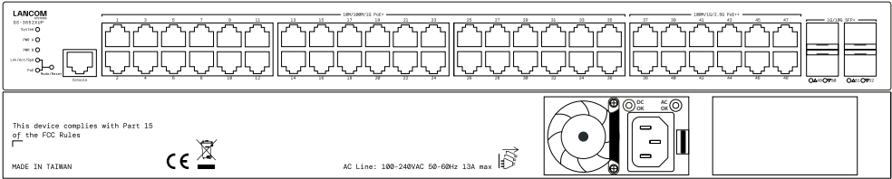
V D LANCOM GS-3652XUP
