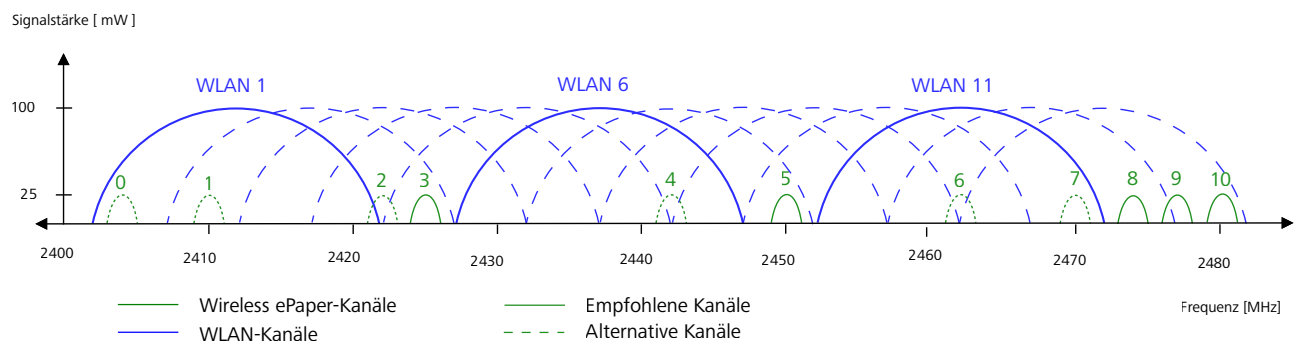
Abbildung 1: Koexistenz von WLAN und Wireless ePaper im 2,4 GHz-Frequenzband
