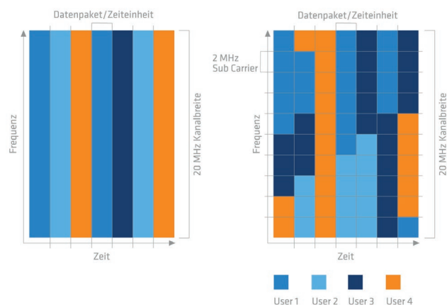
Abb. 3: Vergleich OFDM- vs. OFDMA-Technologie
