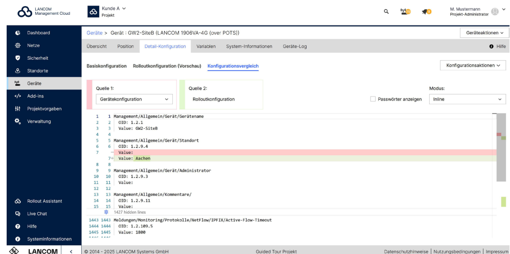
Abbildung 2: Konfigurationsvergleich
