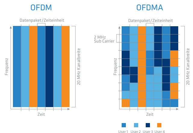
Abb. 1: Vergleich OFDM- (Wi-Fi 5) vs. OFDMA-Technologie (Wi-Fi 6)
