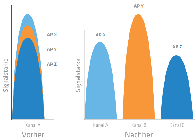
Abb. 1: Kanalverteilung durch Managed RF Optimization
