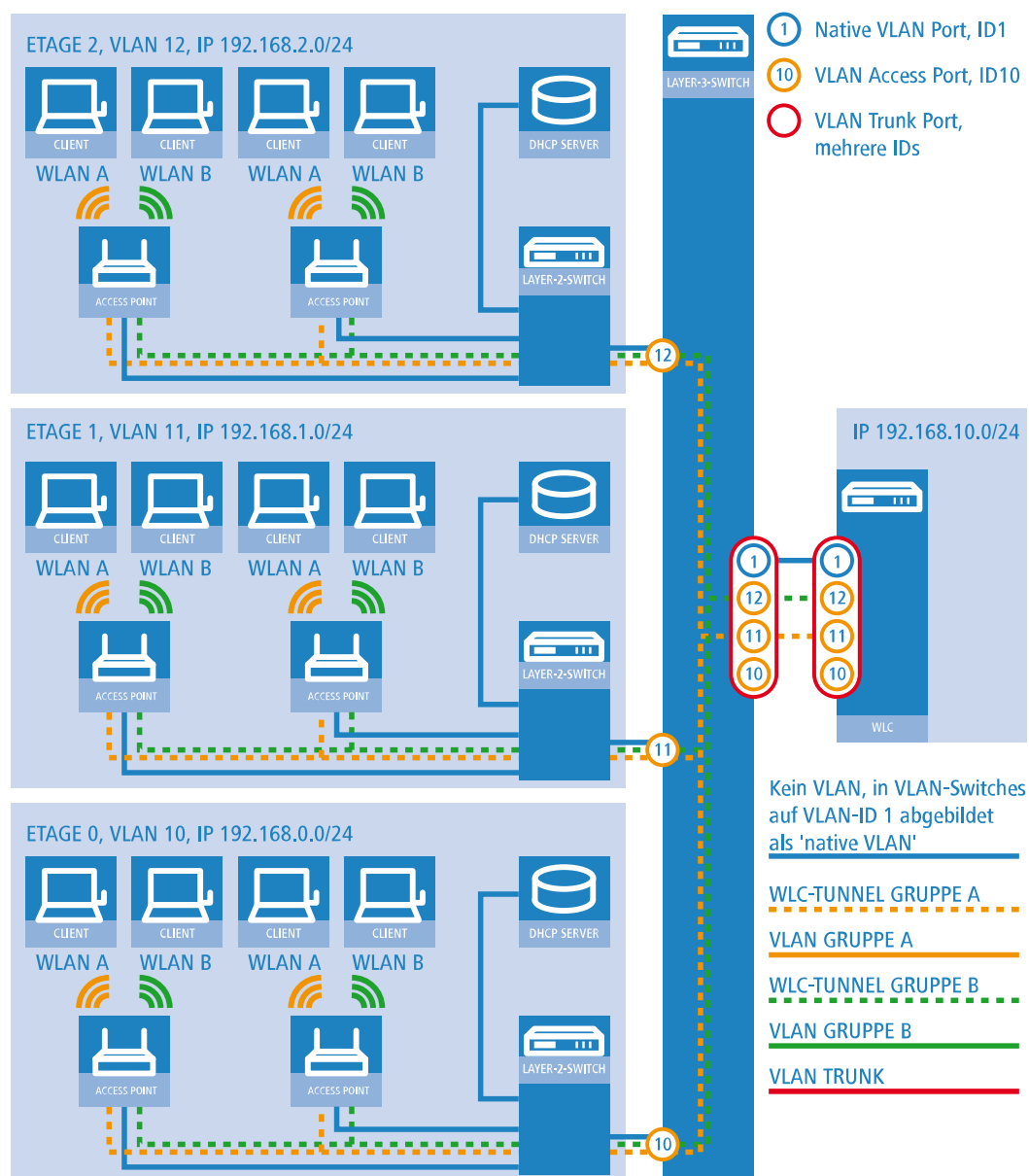
Abbildung 3: Anwendungsbeispiel Layer-3-Roaming
