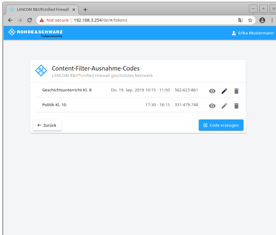
Abbildung 4: Ausnahme-Code: Managementmodus
