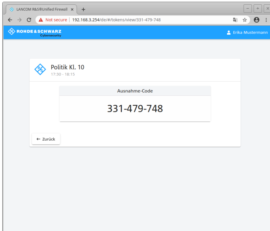
Abbildung 3: Ausnahme-Code: Präsentationsmodus
