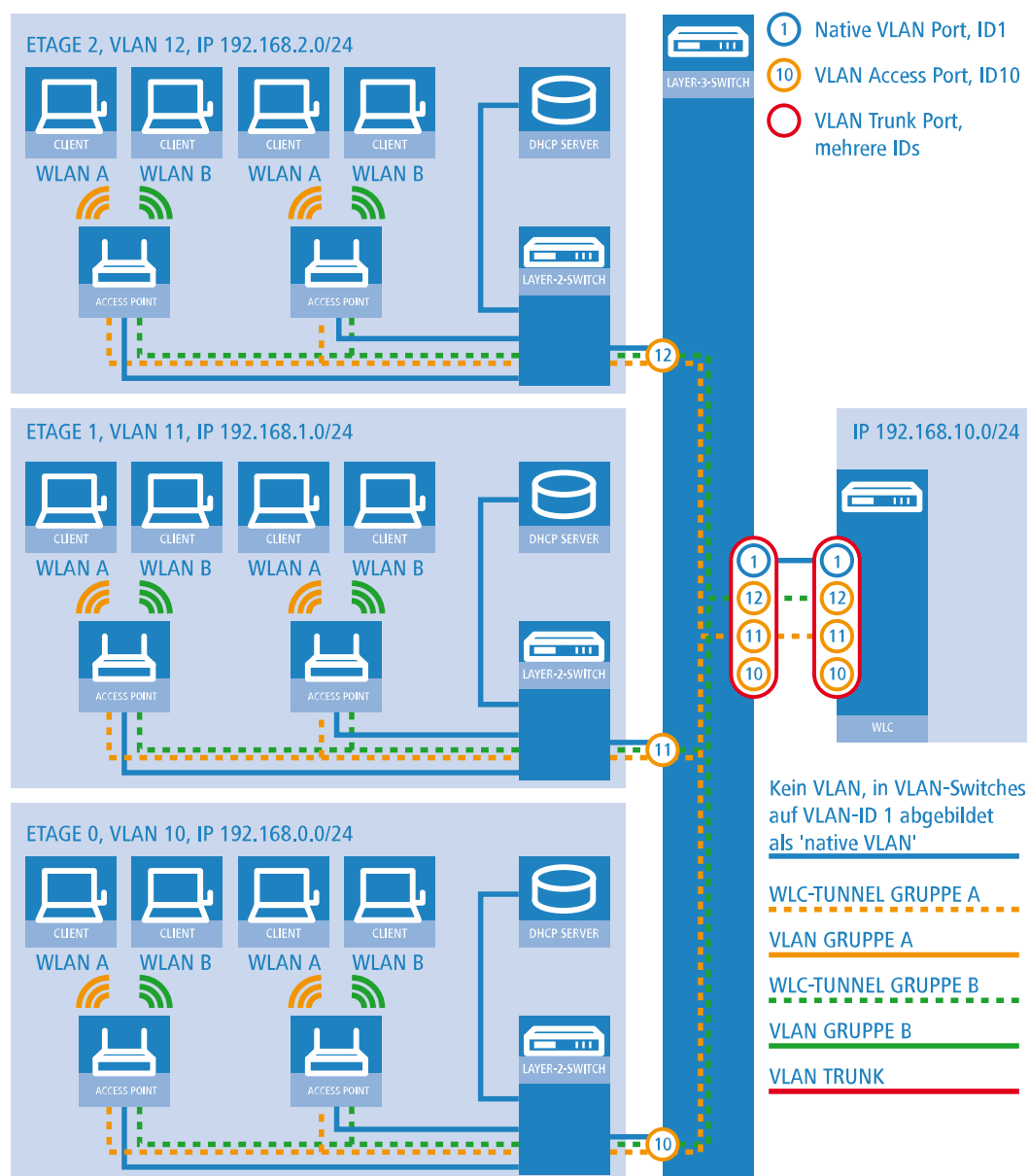
Abbildung 8: Anwendungsbeispiel Layer-3-Roaming
