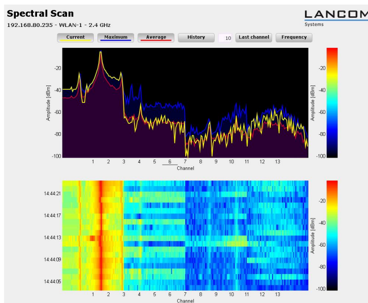
Abbildung 2: Spectral Scan, Kanal-Anzeige Current, Maximum, Average, Störung durch Funk-Kamera
