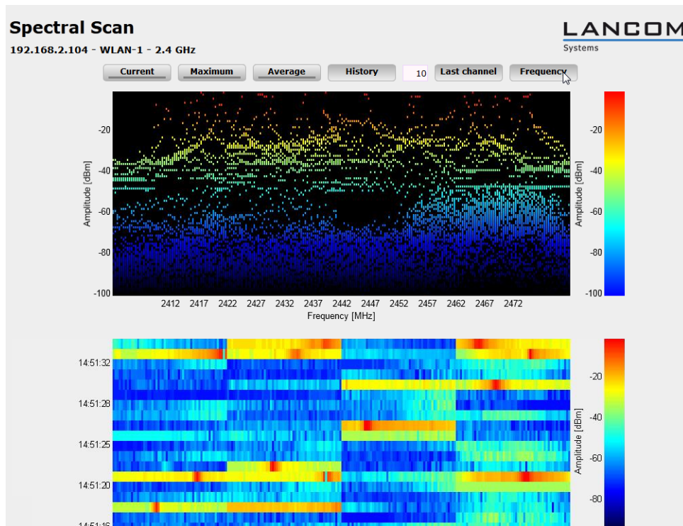
Abbildung 1: Spectral Scan, Frequenz-Anzeige der letzten 10 History-Werte
